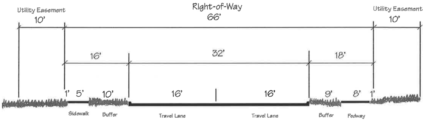
Major Collector 'Option A'
